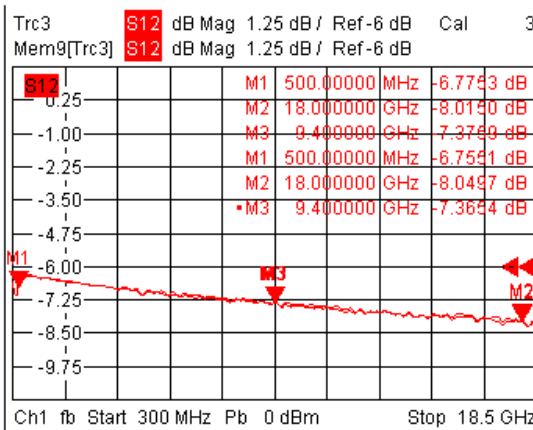
插损及幅度平衡
