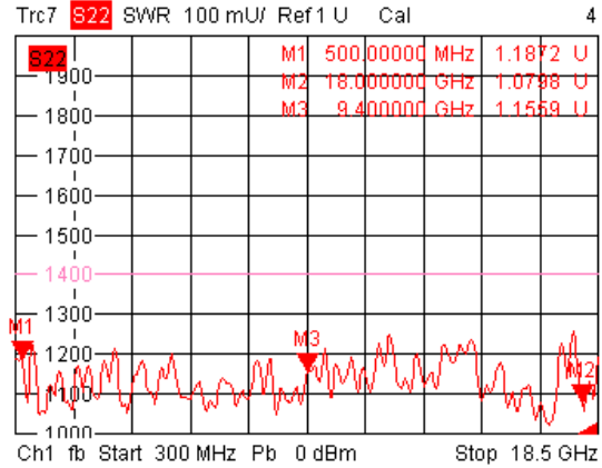
输出驻波比
