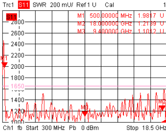
输入驻波比
