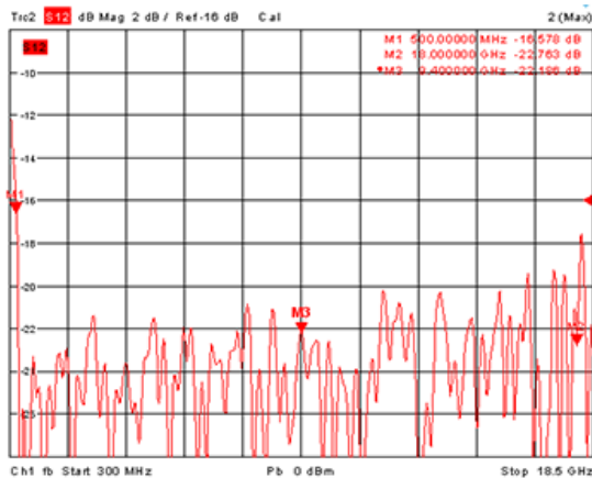
隔离度
