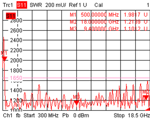
Input VSWR
