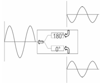
差分-单端信号变换
