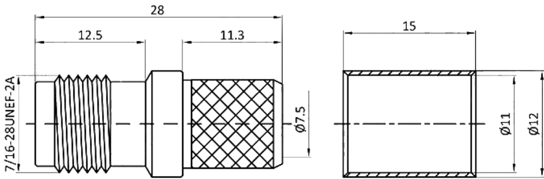
结构尺寸图（单位：mm） 误差±1%
