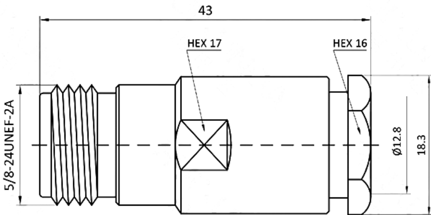
结构尺寸图（单位：mm） 误差±1%
