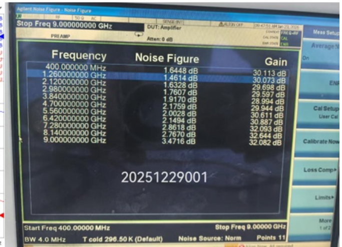
噪声系数曲线
