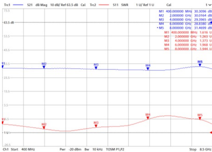
增益曲线
