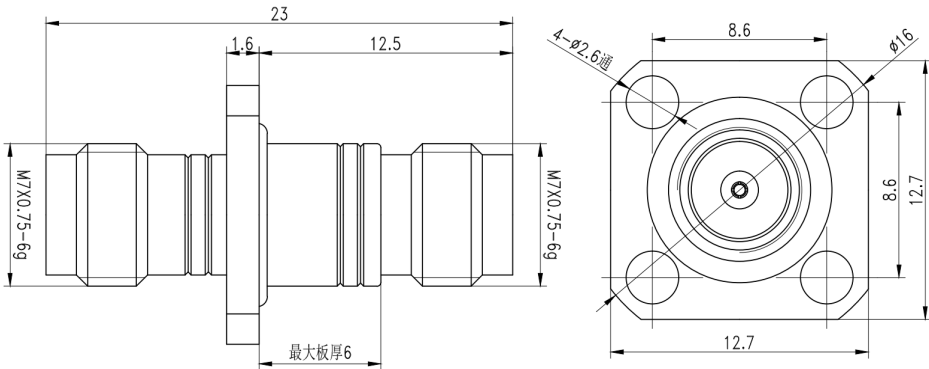
结构尺寸图（单位：mm） 误差±1%
