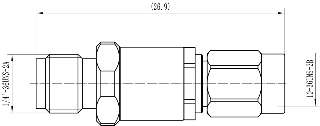
结构尺寸图（单位：mm） 误差±1%
