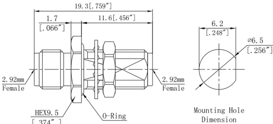
结构尺寸图（单位：mm） 误差±1%
