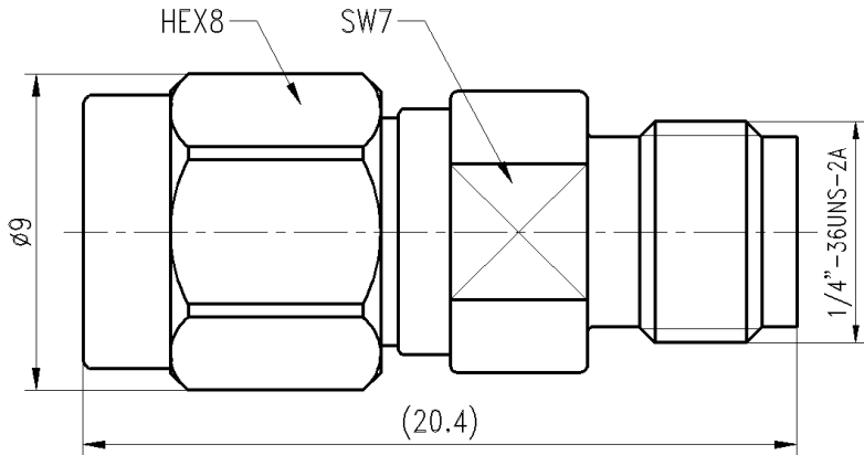
结构尺寸图（单位：mm） 误差±1%
